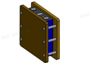
Fig. 2 Schematic diagram of clamp for cell testing 图2 电芯测试夹具示意图
